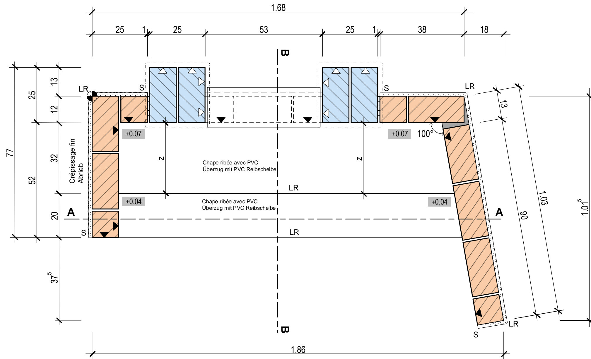
VUE EN PLAN (G-G) GRUNDRISS (G-G)
