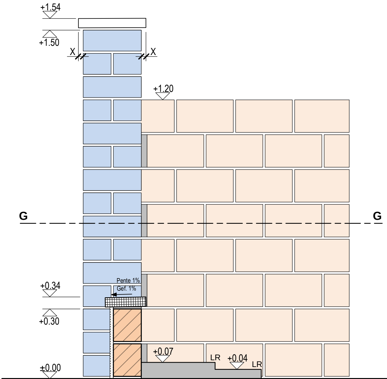
COUPE B-B SCHNITT B-B
