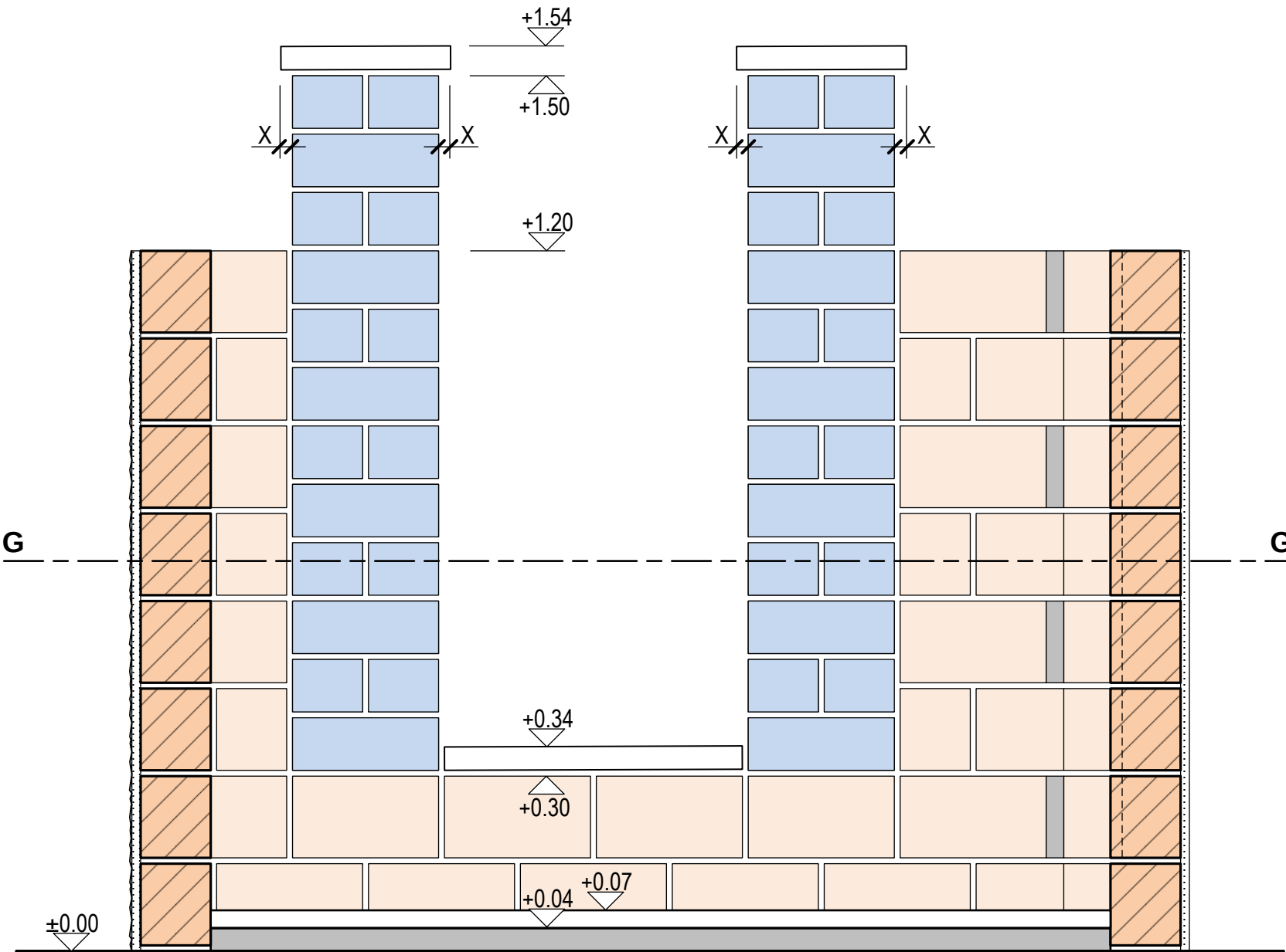
COUPE A-A SCHNITT A-A
